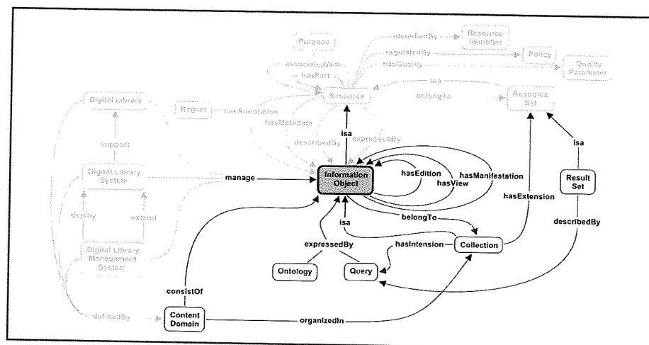
Figura 9. Mappa concettuale del dominio Content
