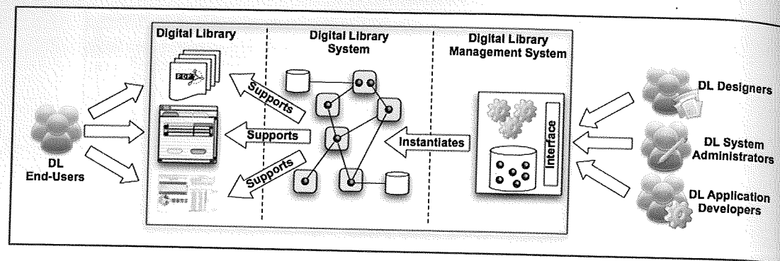
Figura 4. I ruoli principali degli attori rispetto alla struttura a tre livelli
