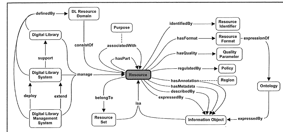
Figura 8. Mappa concettuale del dominio DL Resource 31
