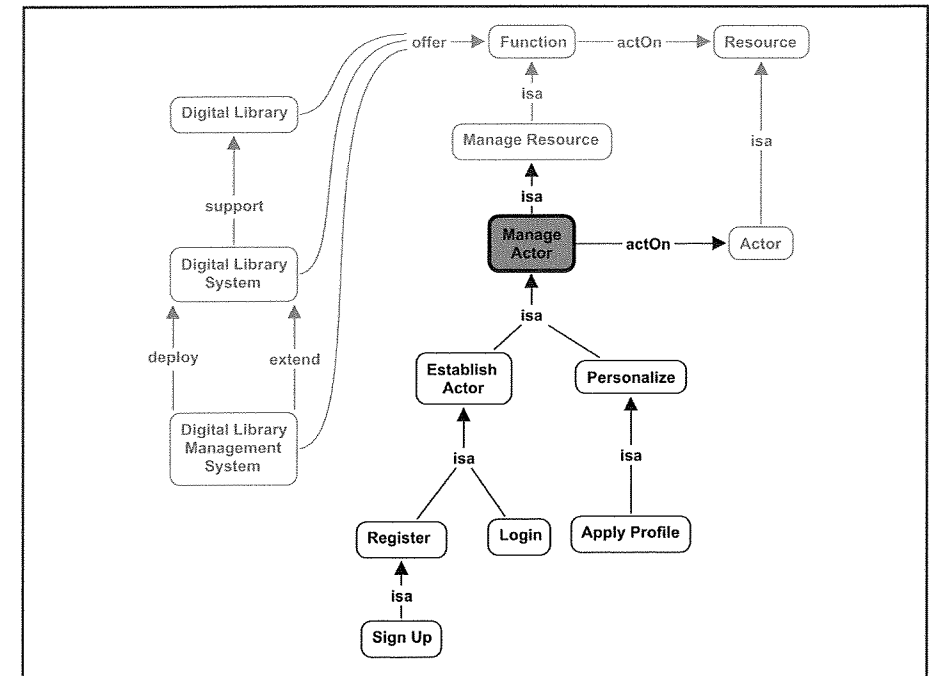
Figura 16. Mappa concettuale di Manage Actor Functions
