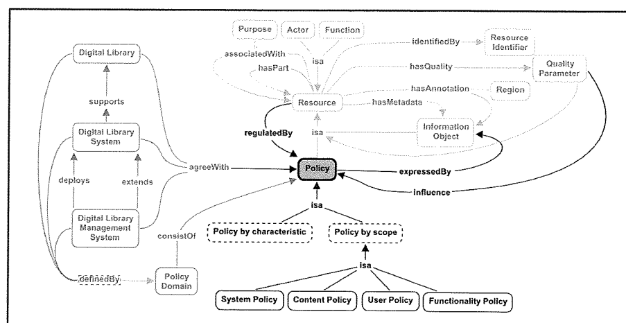
Figura 20. Mappa concettuale del dominio Policy
