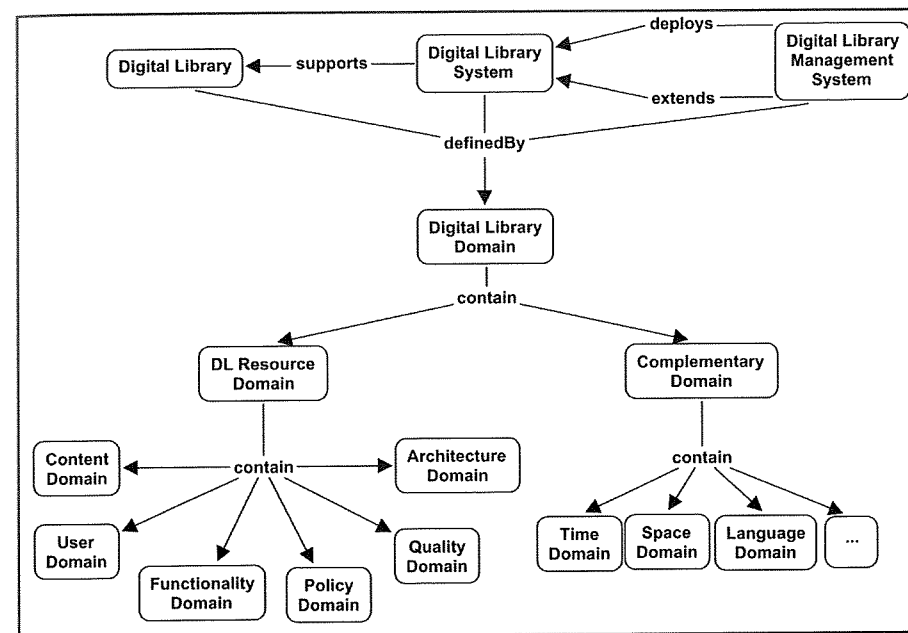
Figura 7. Mappa concettuale dei domini delle biblioteche digitali
