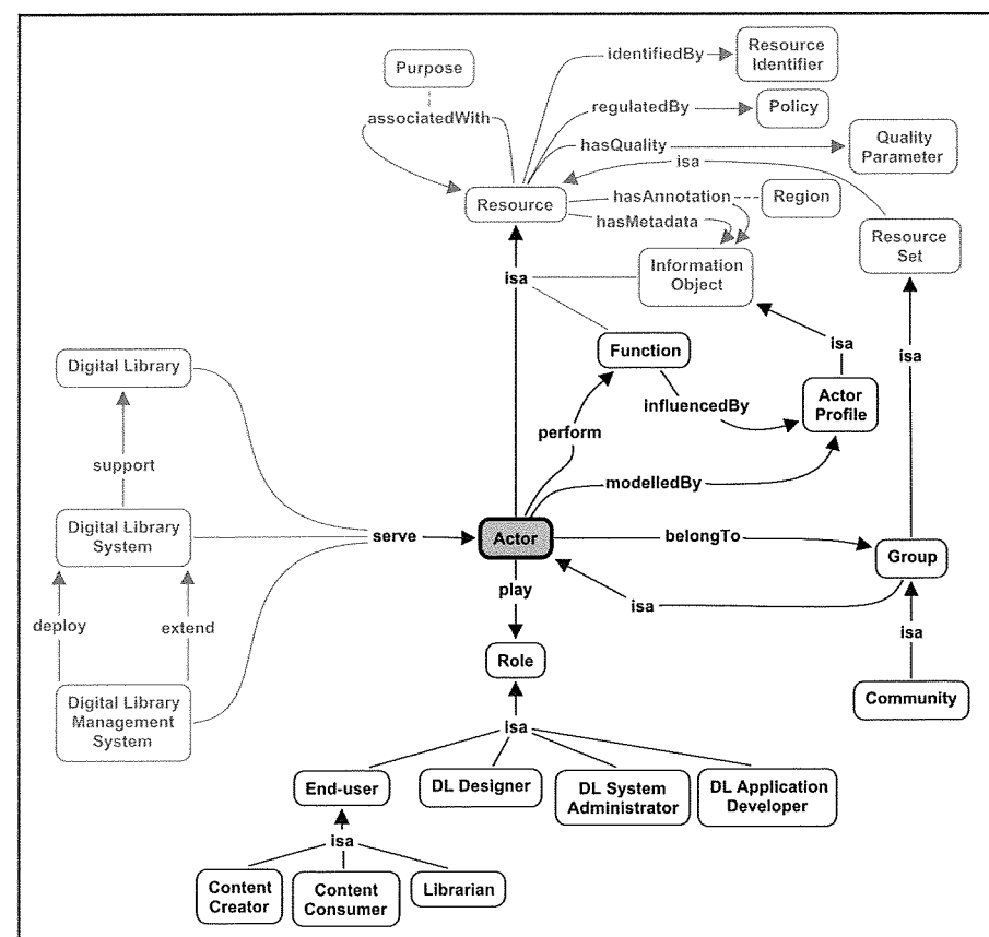
Figura 10. Mappa concettuale del dominio User
