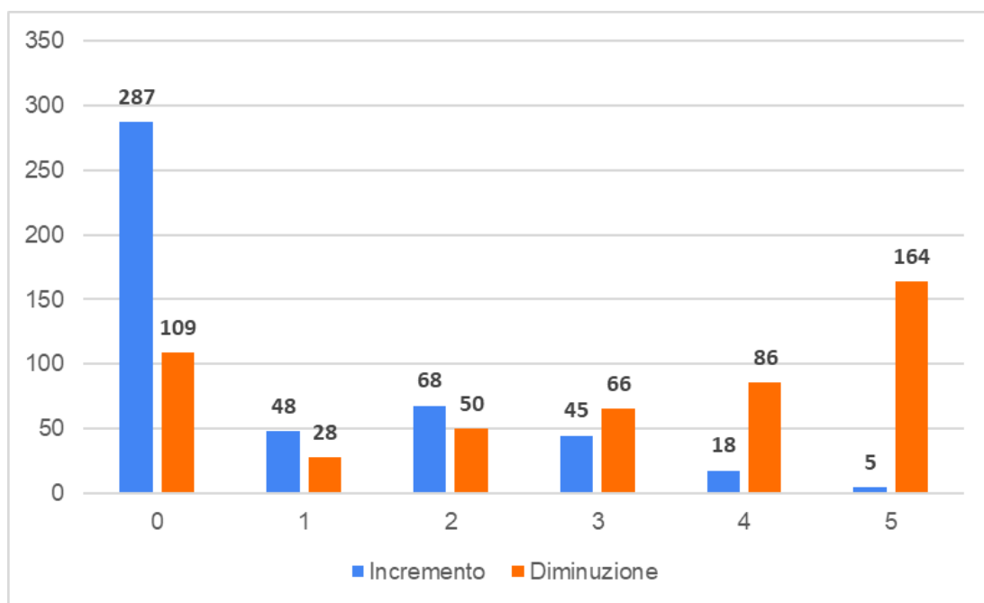
Grafico 14 - Misurazione Lending
