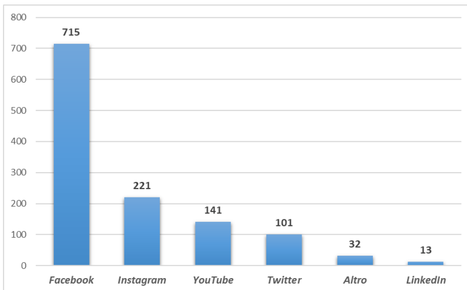
Grafico 23 - Canali social
