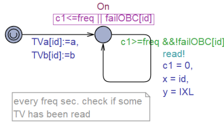
Fig. 15. The OBC_VT automaton
