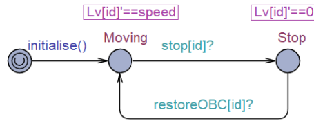
Fig. 12. The OBC_Drive automaton
