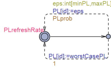
Fig. 10. The OBC_PL automaton
