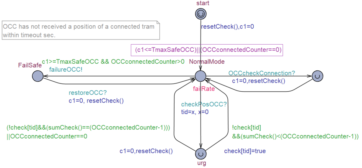
Fig. 7. The OCC_Supervision automaton
