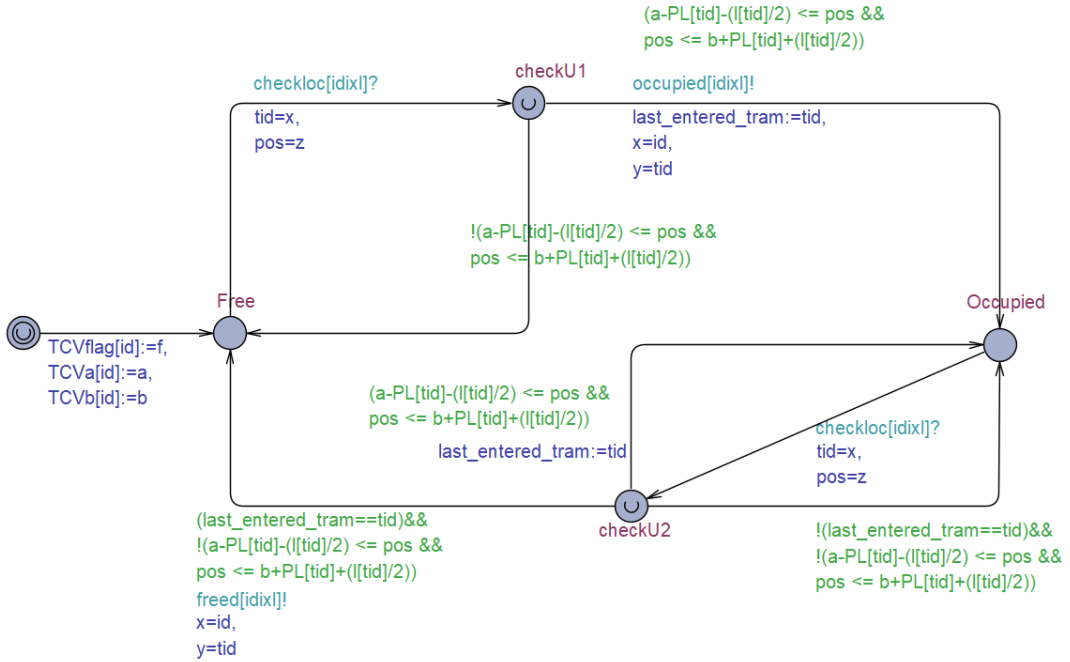
Fig. 22. The IXLVTC automaton.
