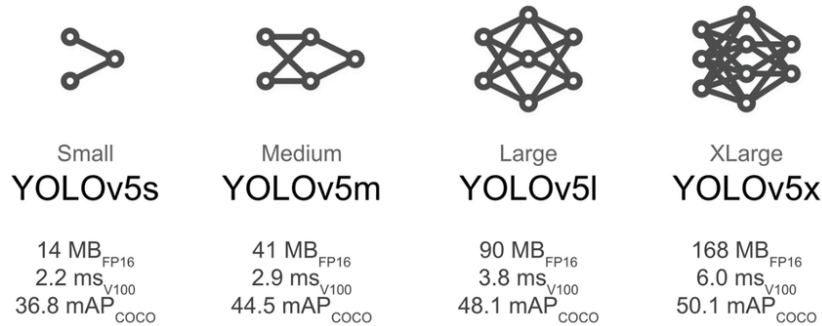
Figure 13: Confronto tra i diversi modelli YOLOv5 (Fonte immagine: [15]).
