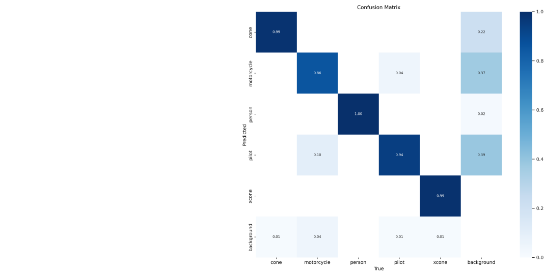
Figure 39: La matrice di confusione del modello con yolov5m
