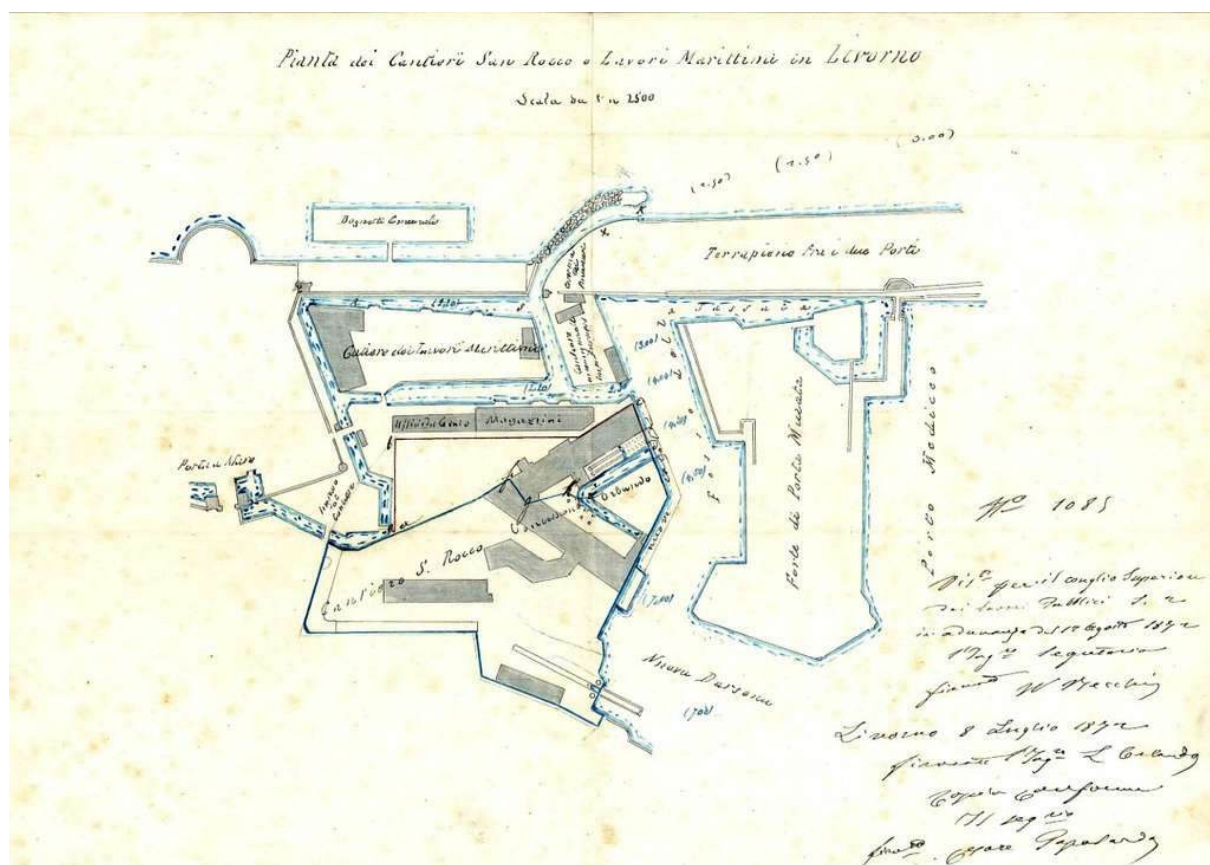
Figura 2. “Planimetria del Cantiere navale Fratelli Orlando comprendente i Cantieri San Rocco e Lavori Marittimi”, in Archivio storico del Cantiere navale Luigi Orlando di Livorno , 1872.
