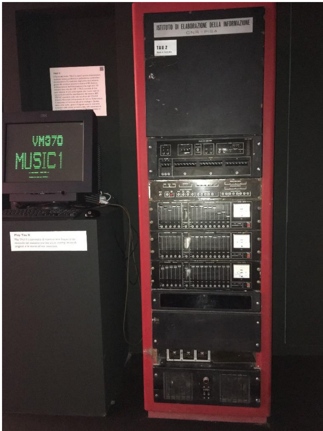
Figura 1: Disposizione del "terminale" accanto all'Unità Digitale del TAU2
