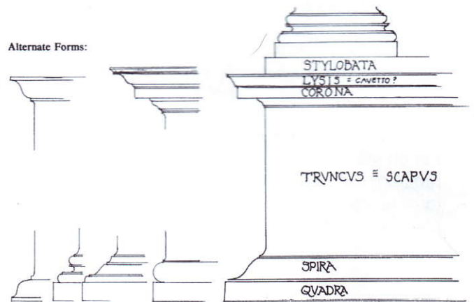
Vitruvius beskrivning av romerska listverk. Från I.D. Rowland och T.N. Howe, Vitruvius Ten Books on Architecture , Cambridge 1999, fig. 45
