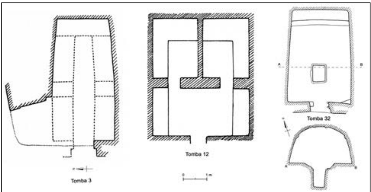
Fig. 4 - Planimetrie delle tombe nn. 3, 12 (da Quilici Gigli 1970, Fig. 9, 3) e 32.
