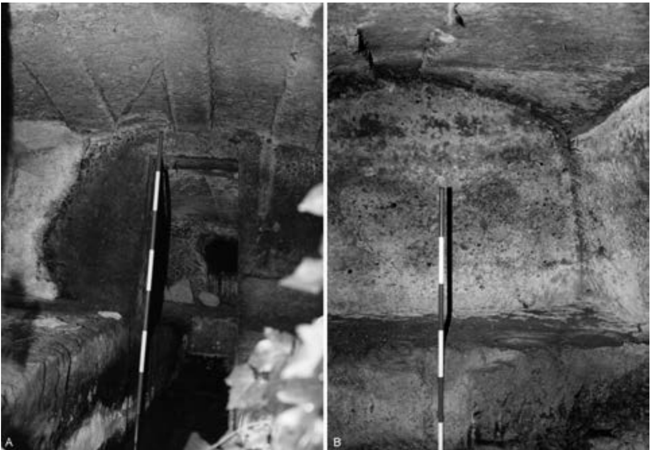
Fig. 16 - La prima camera della tomba n. 82 (A), con soffitto caratterizzato da columen e mutuli a rilievo, e l'interno della tomba n. 87 (B), con columen incassato.
