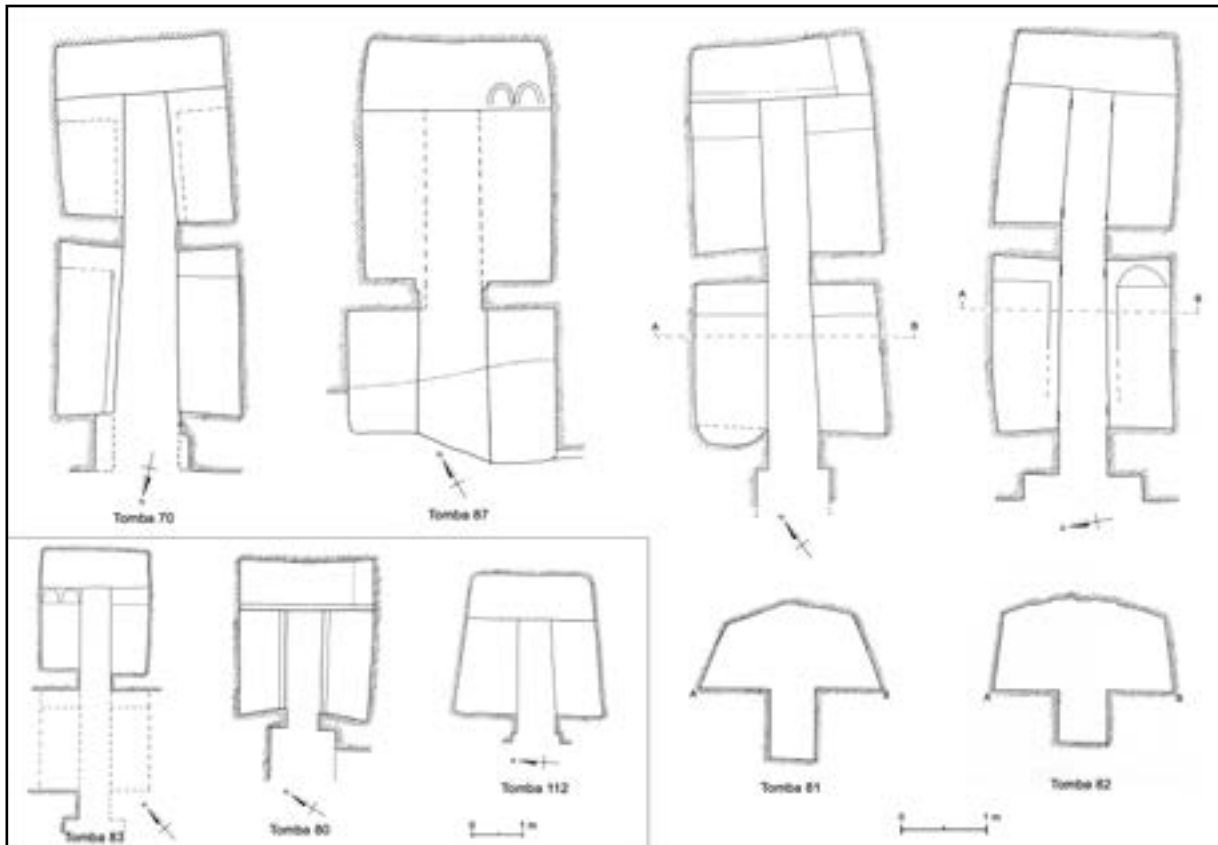
Fig. 13 - Planimetrie delle tombe nn. 70, 80, 81, 82, 83, 87 e 112; delle nn. 81 e 82 compaiono anche le sezioni.
