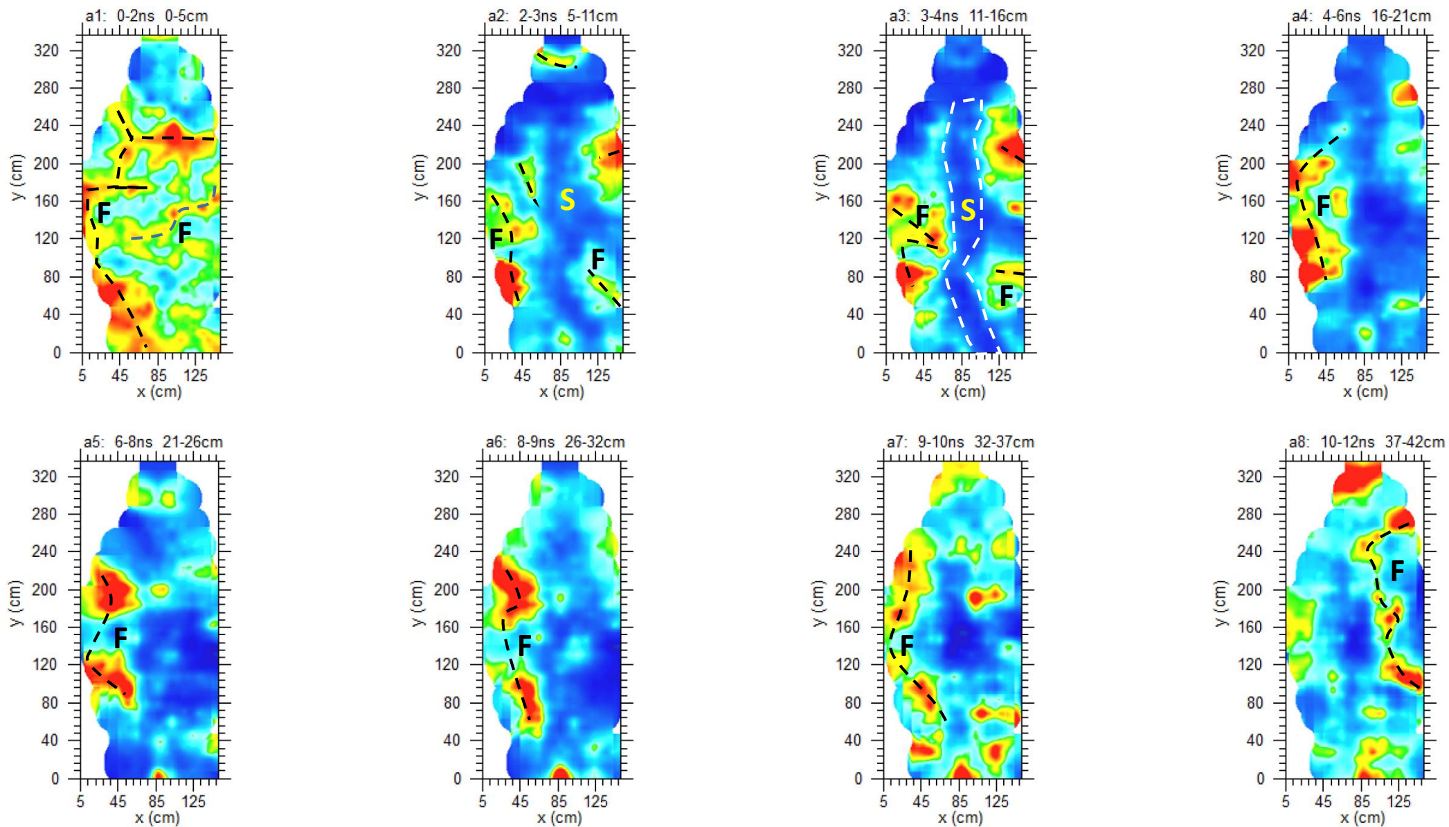
Fig. 20: Statua Liberalitá: antenna da 2 GHz: Depth slices. F: fessura interna; S: strato di diverso materiale.
