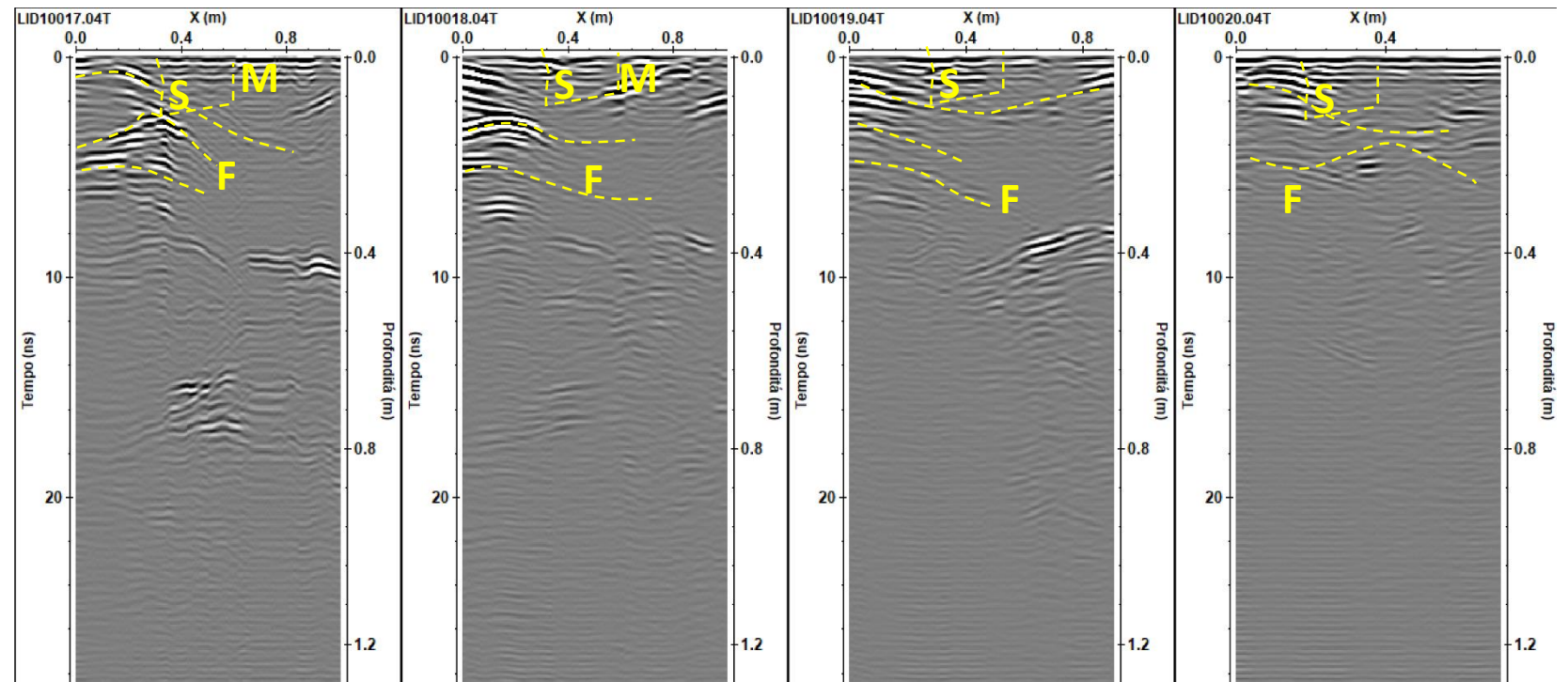
Fig. 15: Statua Liberalità: antenna da 2 GHz: sezioni radar elaborate relative ai profili R17,..., R20. F: fessura interna; S: strato di diverso materiale; M: metallo.
