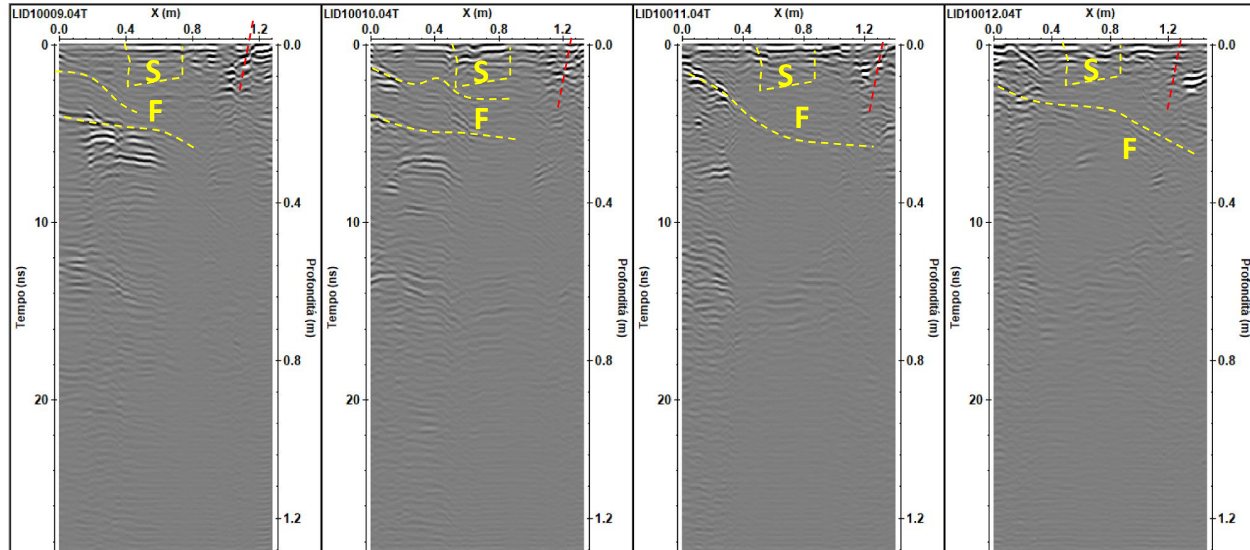
Fig. 13: Statua Libertá: antenna da 2 GHz: sezioni radar elaborate relative ai profili R9,..., R12. F: fessura interna; S: strato di diverso materiale.
