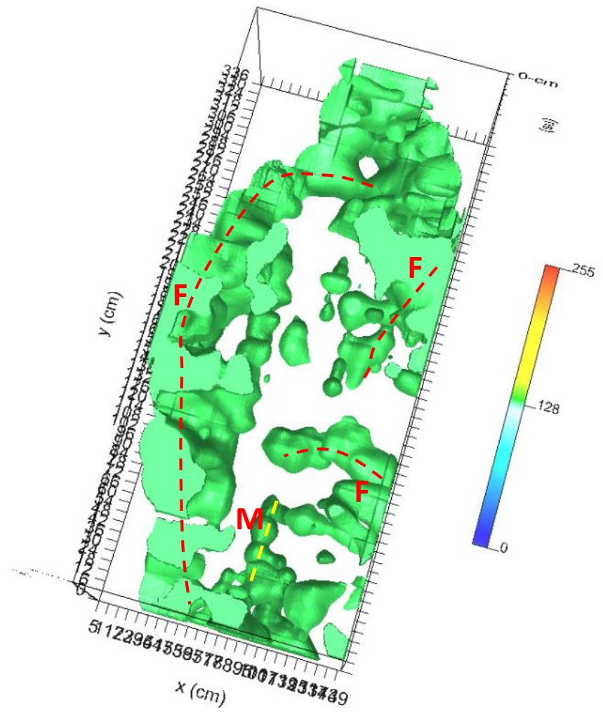
Fig. 21: Statua Liberalità: antenna da 2 GHz: Isosuperficie di ampiezza dell'onda elettromagnetica. F: fessura interna; M: metallo.
