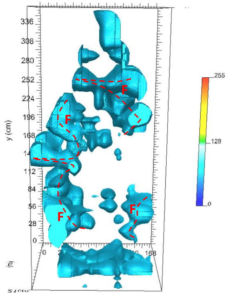
Fig. 9: Statua Libertá: antenna da 900 MHz: Isosuperficie di ampiezza dell'onda elettromagnetica. F: fessura interna.
