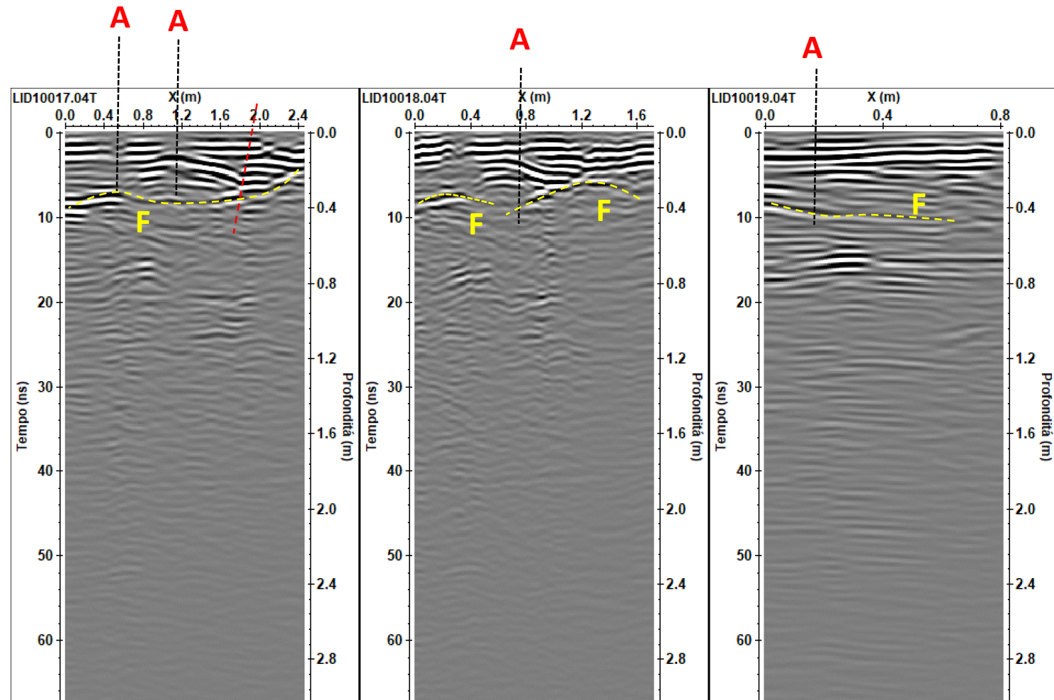
Fig. 7: Statua Liberalità: antenna da 900 MHz: sezioni radar elaborate relative ai profili R17,..., R19. F: fessura interna; S: strato di diverso materiale; M: metallo; A: punti di divisione dei blocchi
