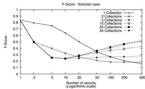
Figure 15. ScienceI case: F1 values.
