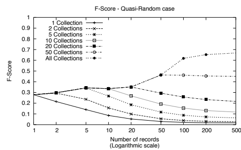
Figure 17. Quasi-random case: F1 values.
