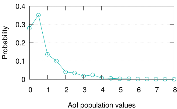
(a) PDF of K_t(r)
