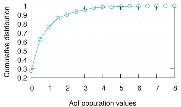
(b) CDF of K_t(r)
