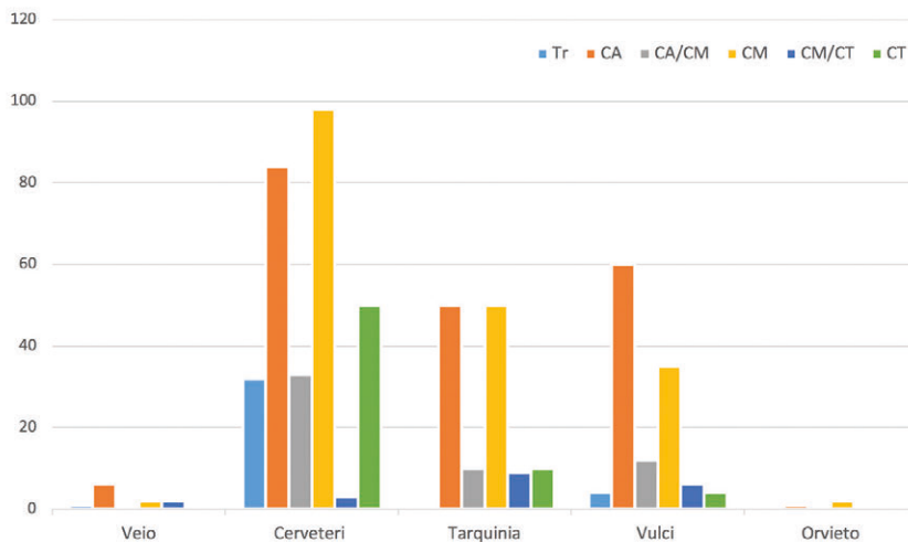
Fig. 9. Grafico finale.
